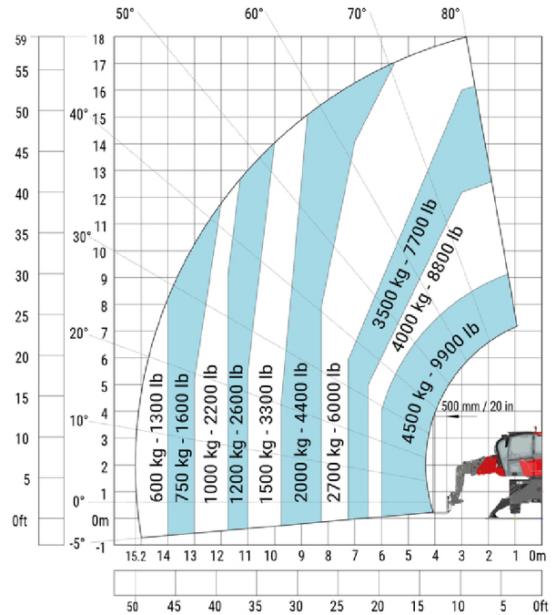
Rotazione su stabilizzatori con forche
